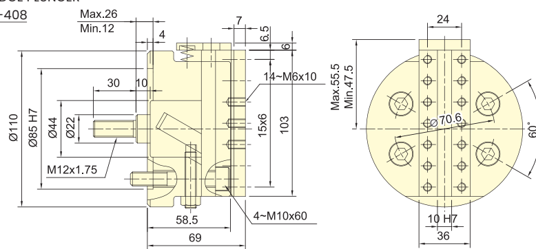
單斜楔式傳動 WEDGE PLUNGER FA-408
